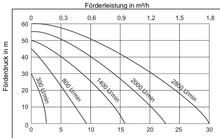
UNISTAR 2000-A mit Frequenzumrichter
