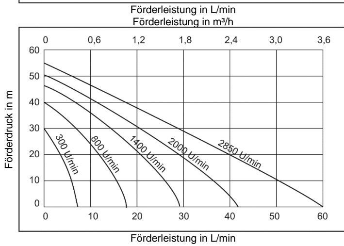
UNISTAR 2000-B mit Frequenzumrichter
