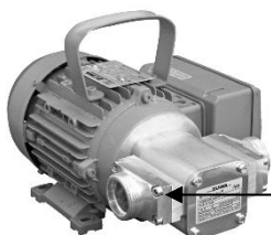
seitl. Anschlussflansch
